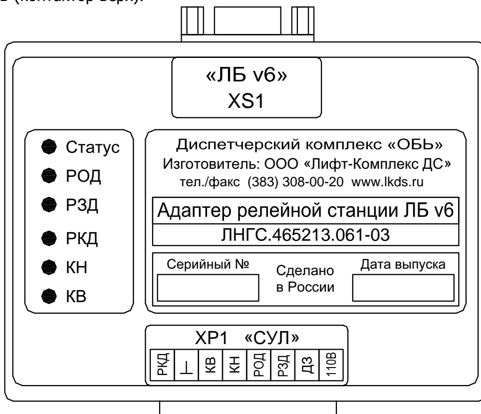
Рис. 2. Внешний вид адаптера релейной станции
